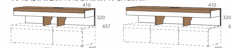
PZ-TVN5 (1 KLOPNA VRATA / POKLOPNA VRATA / FLAP DOOR) PZ-TVN6 (1 KLOPNA VRATA / POKLOPNA VRATA / FLAP DOOR)
