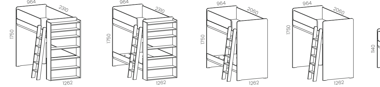
MLRZD, MLRZL na sliki je D izvedba / na sliki je D izvedba /the picture shows R version MLRKD, MLRKL na sliki je D izvedba / na sliki je D izvedba /the picture shows R version MLK MLZ MLV
